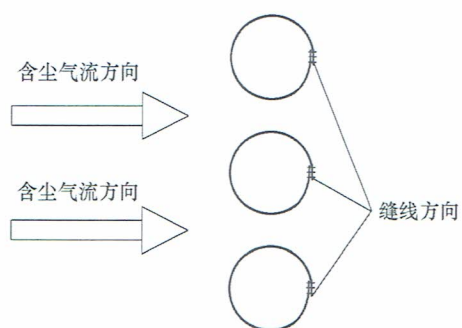
图C.2 滤袋正确的安装位置
