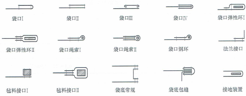
图B.1 外滤式滤袋袋口、袋底缝制形式
